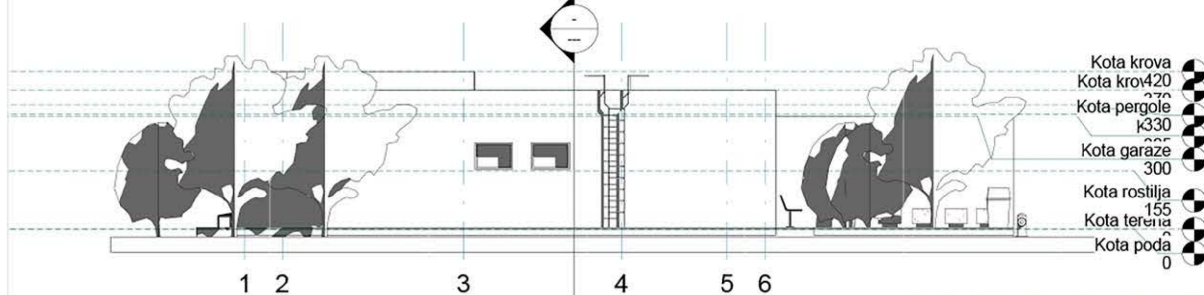
Izgled 4_ Zapadna fasada R 1:100
