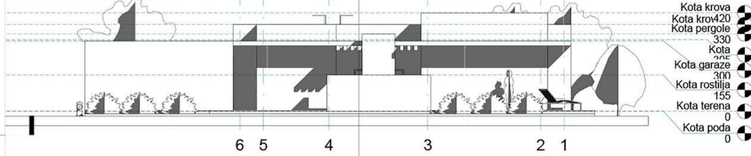
Izgled 3_ Istočna fasada R 1:100
