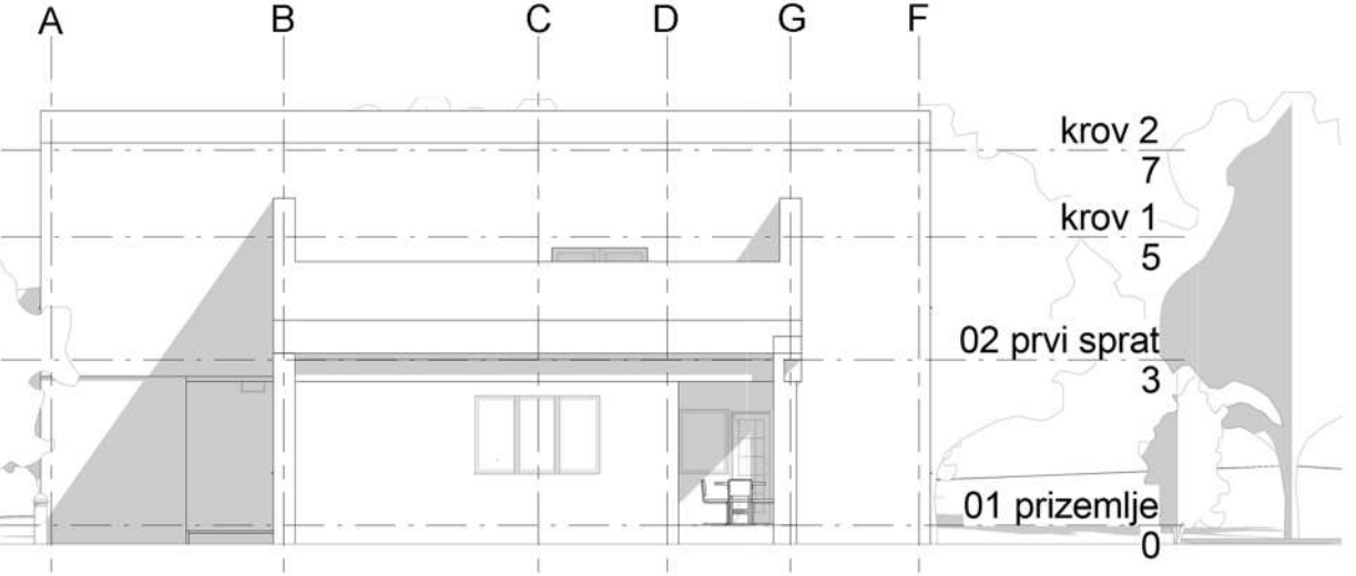
Istočna fasada R 1:150
