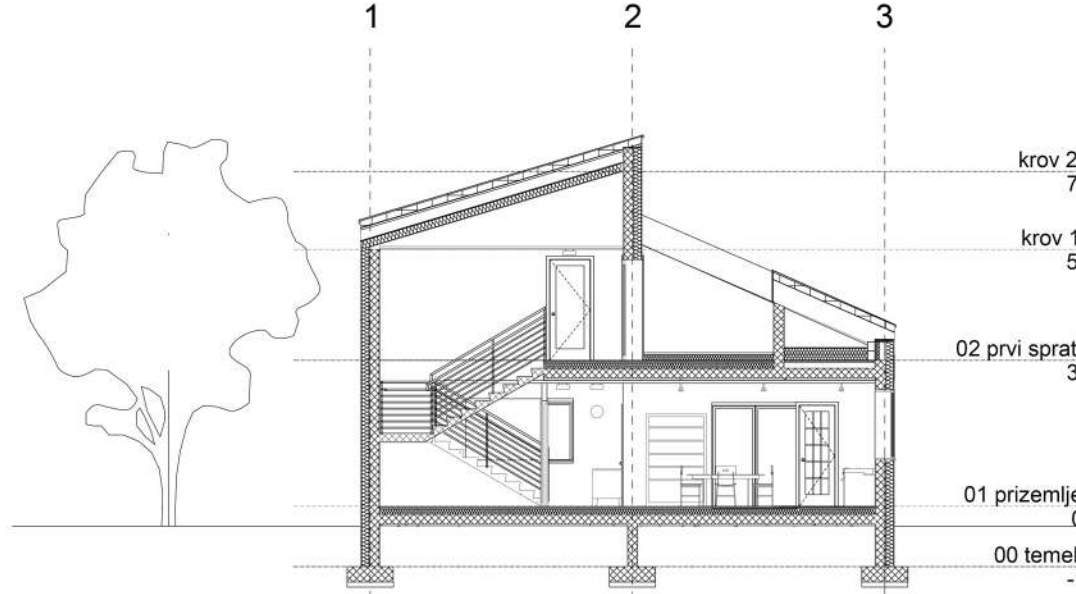
Presek 1-1 R 1:150
