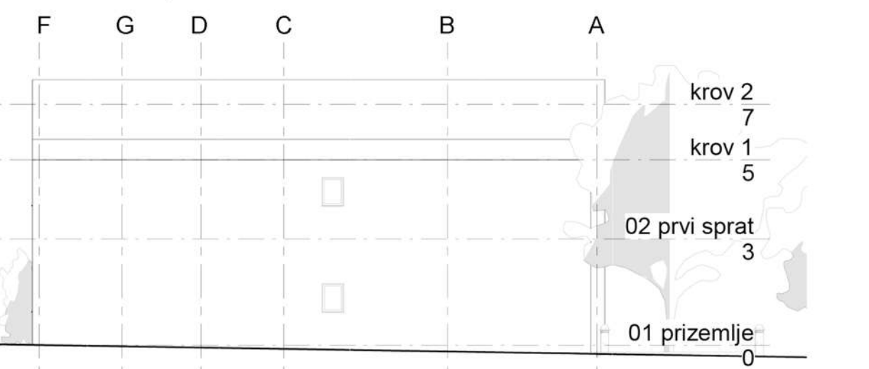
Zapadna fasada R 1:150
