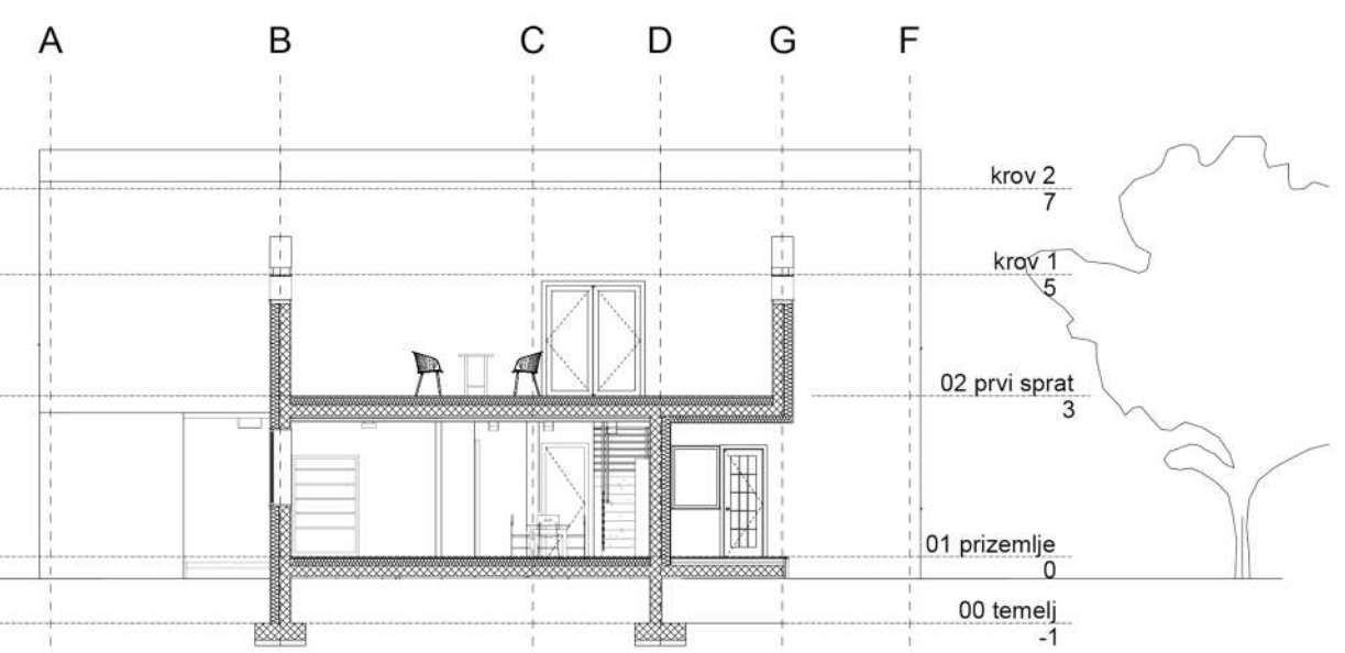
Presek 2-2 R 1:150
