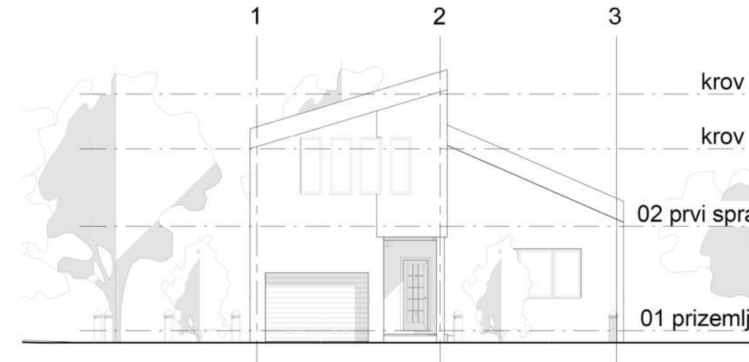
Južna fasada R 1:150
