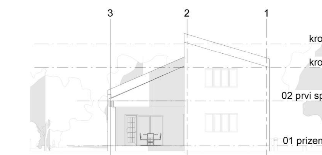
Severna fasada R 1:150
