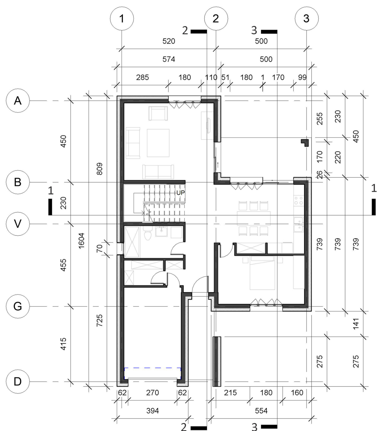
osnova prizemlja
