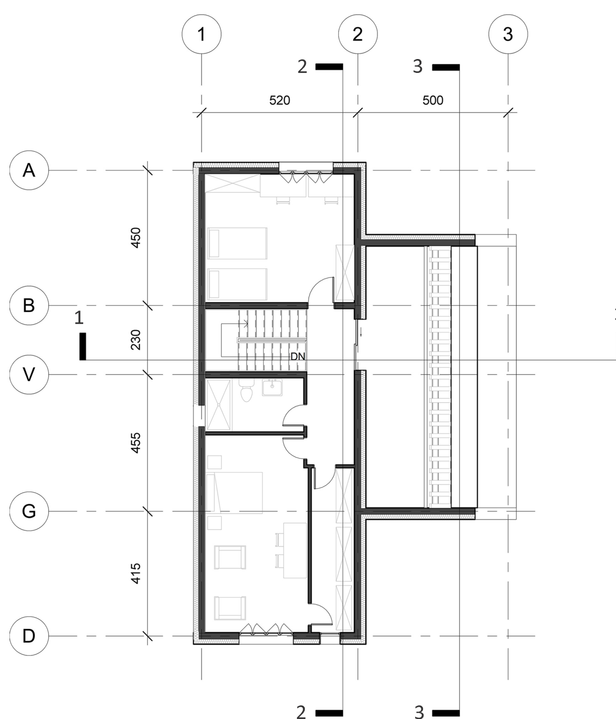
osnova sprata
