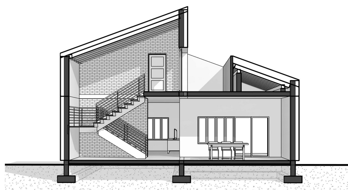
vertikalni presek 1-1
