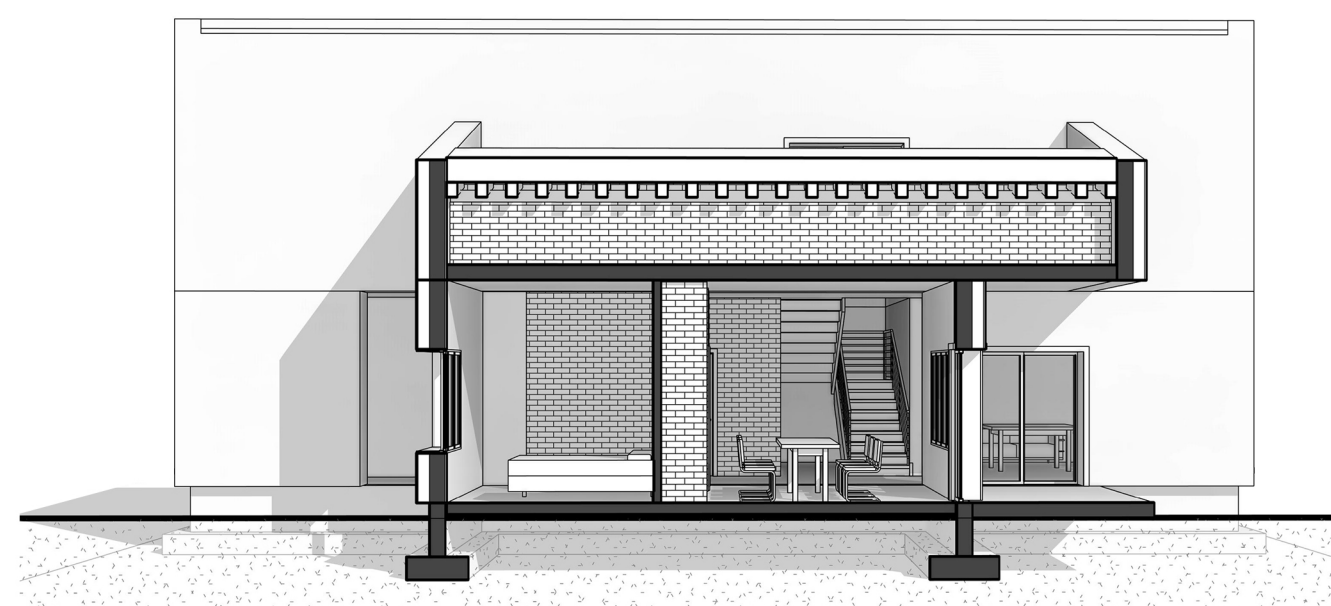
vertikalni presek 2-2
