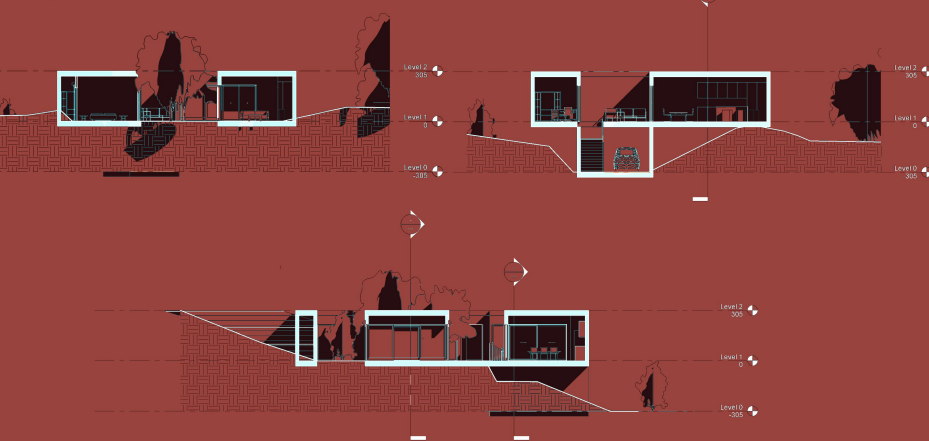
preseci // R_1:200
