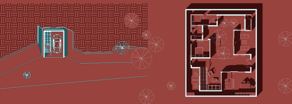
izgledi // R_1:200
