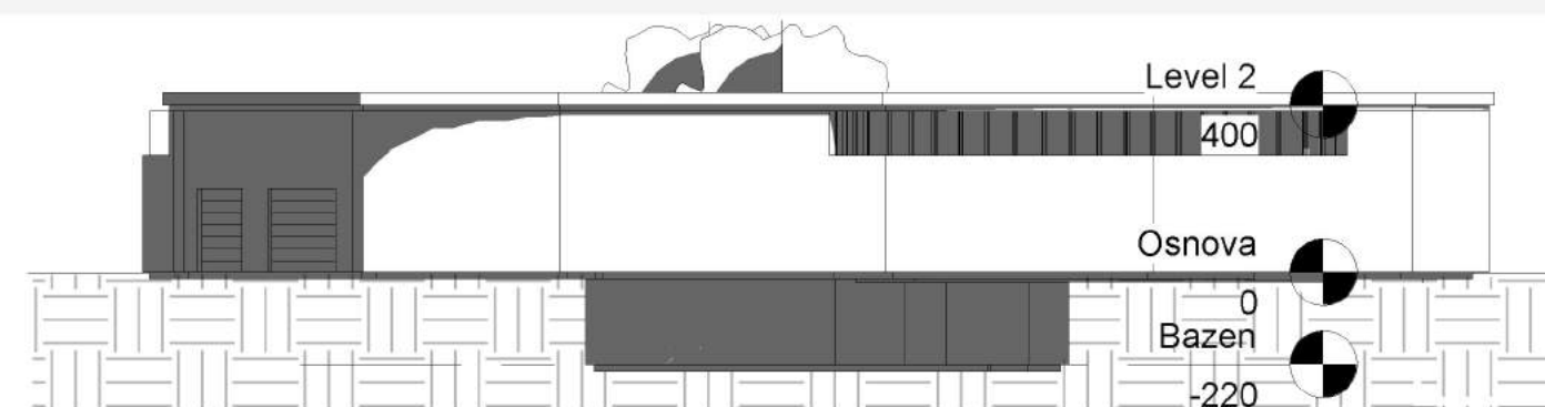
4 Izgled 1 1 : 200
