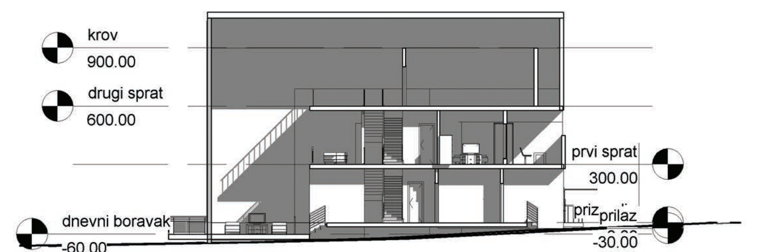
4 Presjek 1 1:200
