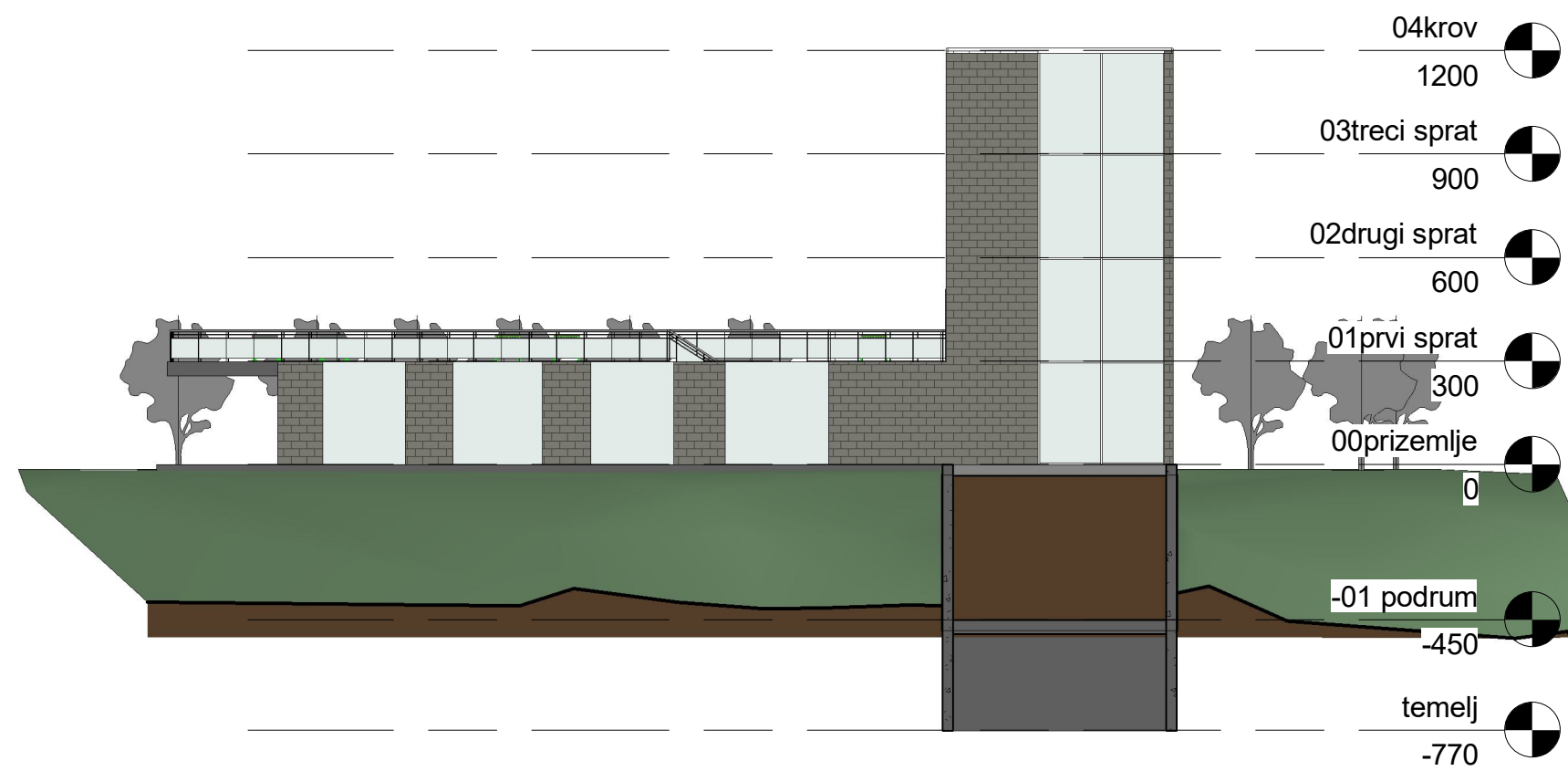
2 North 1 : 200
