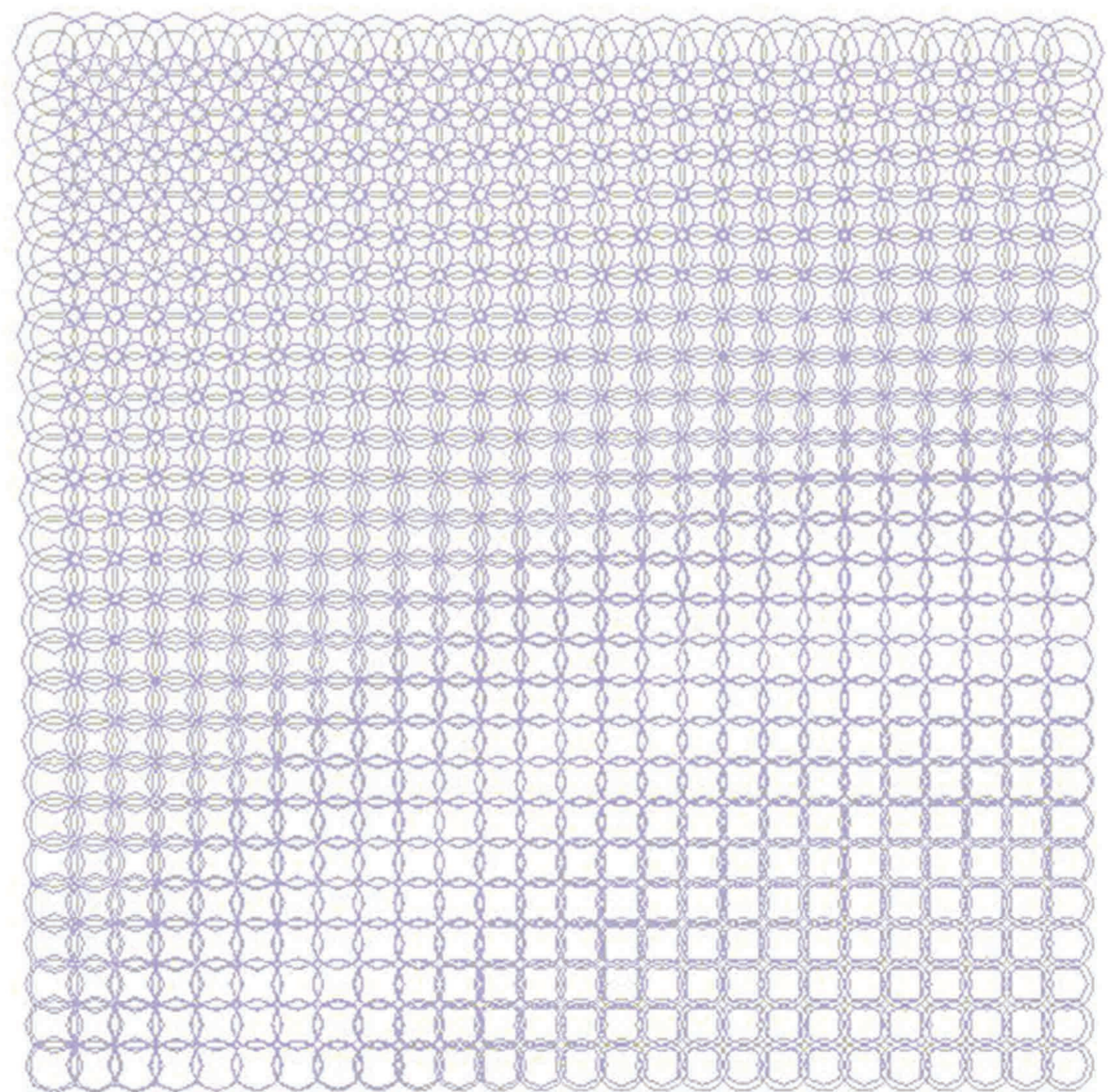
grafička matrica sa aktiviranim atraktorom 2
