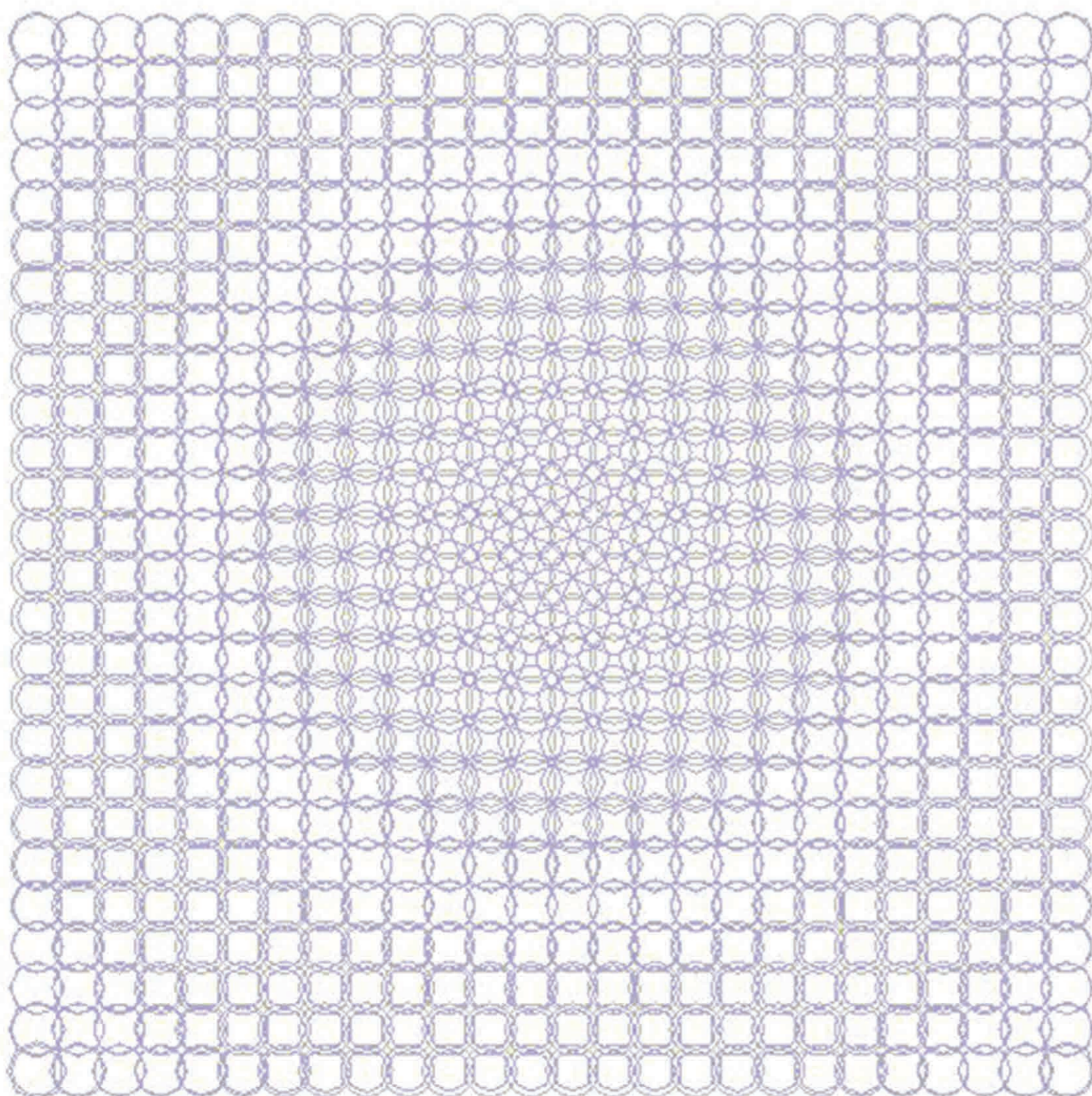
grafička matrica sa aktiviranim atraktorom 1
