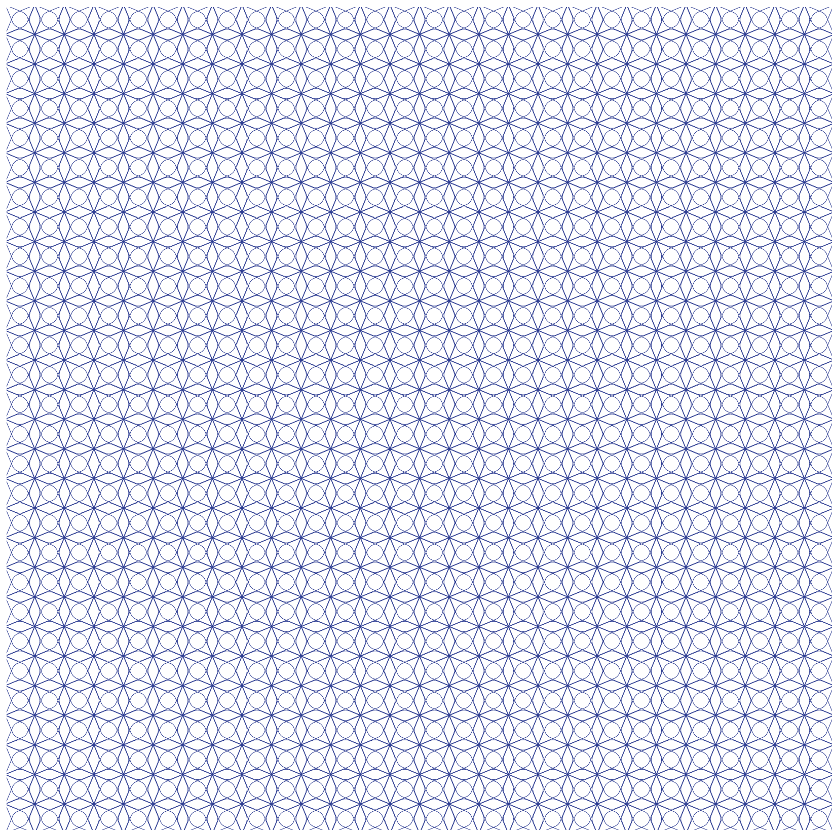
početna matrica
