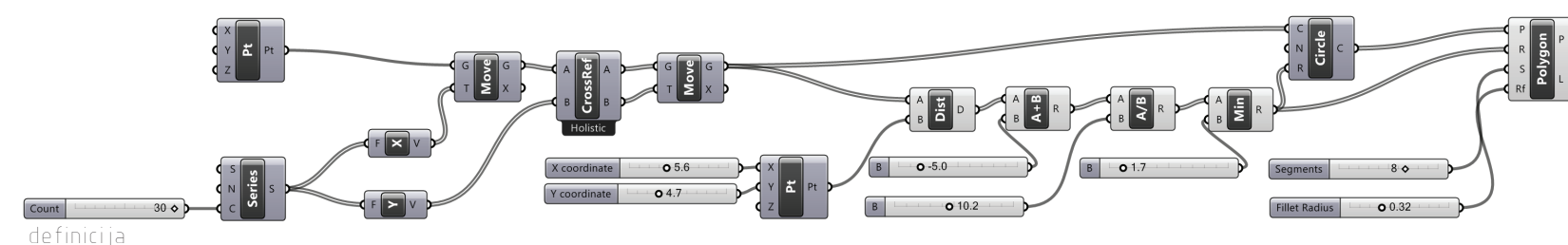
definicija
