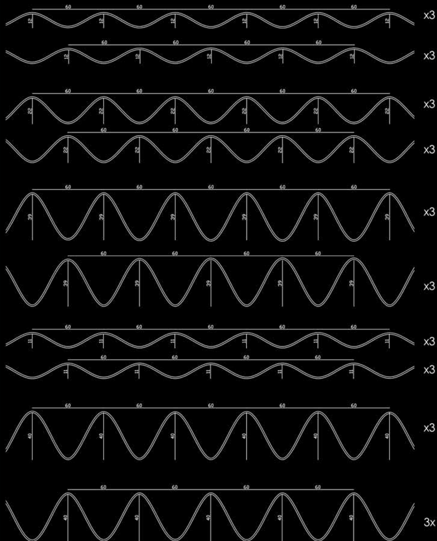
_elementi od žice potrebni za izgradnju ograde
