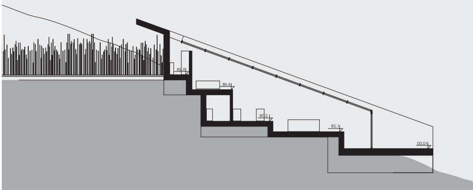
Presek objekta
