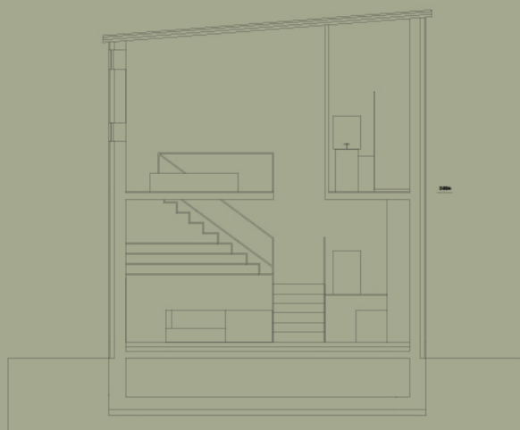
presek A-A
