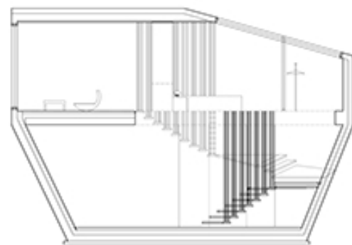
PRESEK
