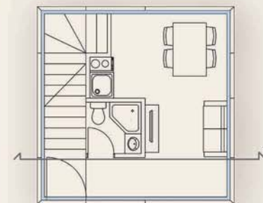
Osnova prizemlja
