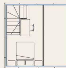
Osnova 1. sprata
