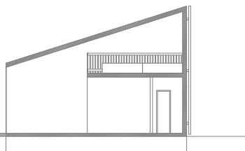
presek 1:1
