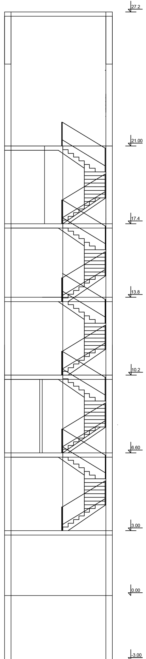
vertikalni preseki R=1:100
