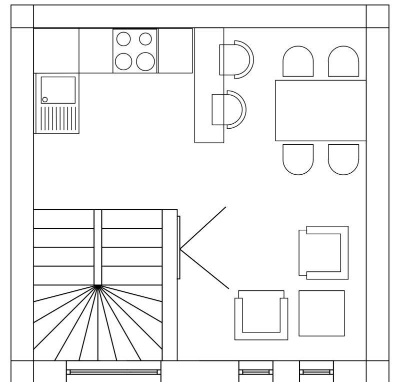
osnova 3 R=1:50
