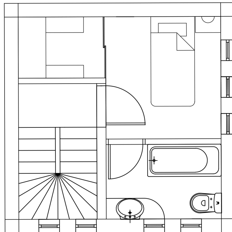
osnova 2 R=1:50
