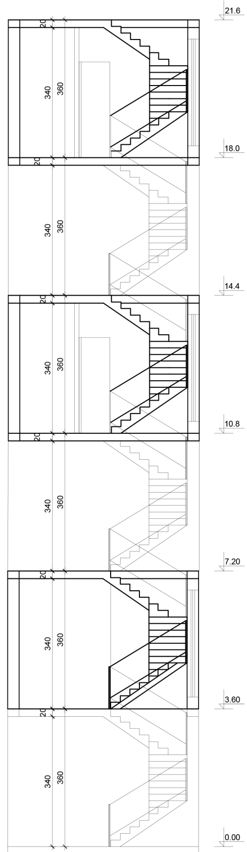
vertikalni presek R=1:100
