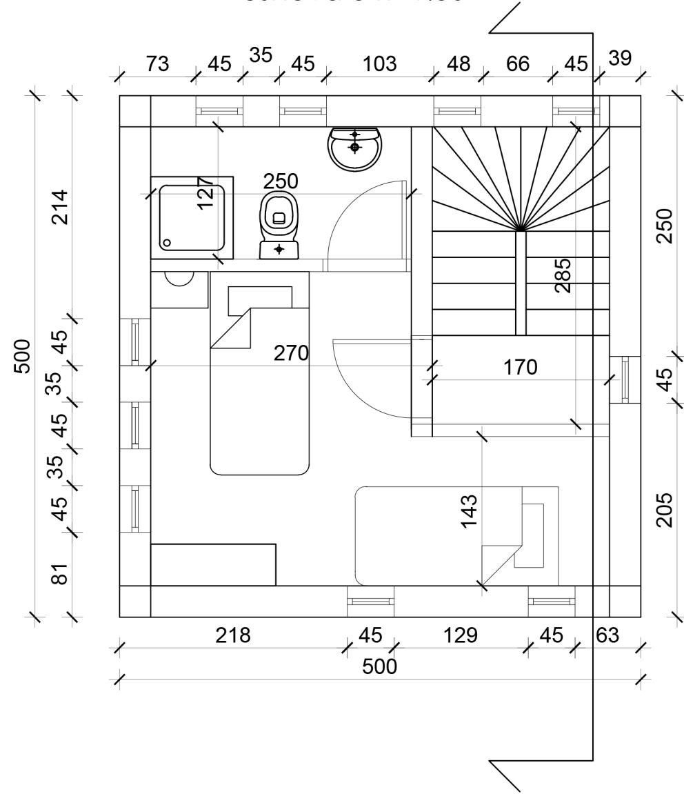
osnova 3 R=1:50
