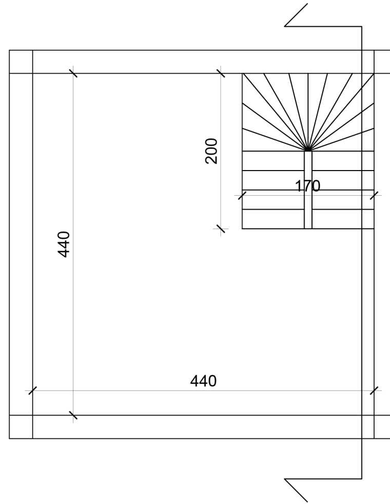
stepenišni prostor R=1:50
