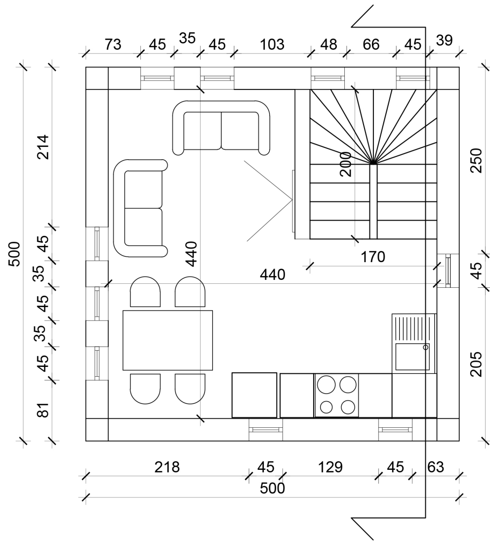
osnova 1 R=1:50
