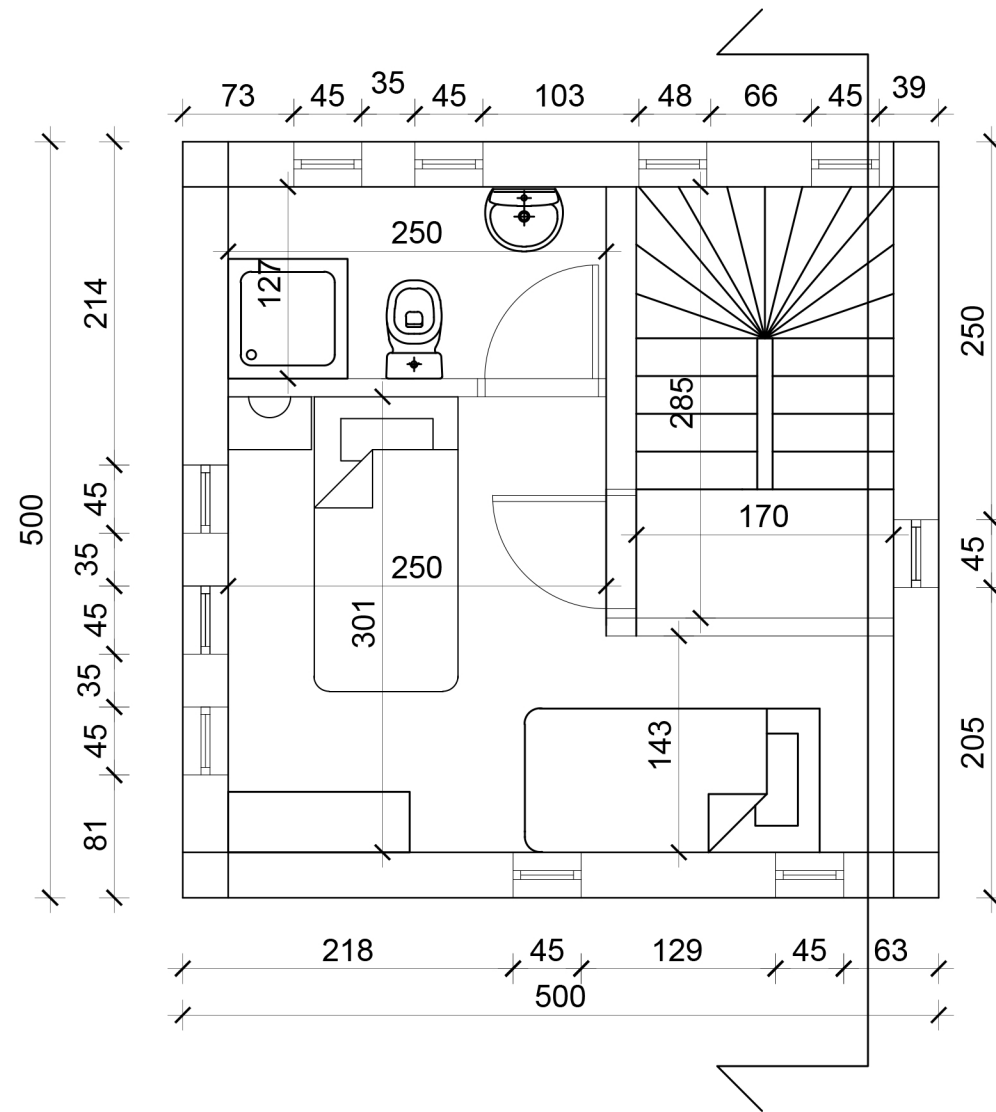
osnova 2 R=1:50
