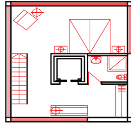
OSNOVA 1. ETAZE R 1 : 50
