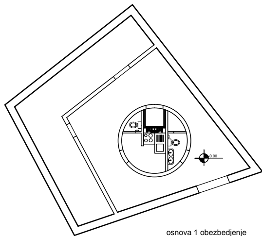
osnova 1 obezbedenje
