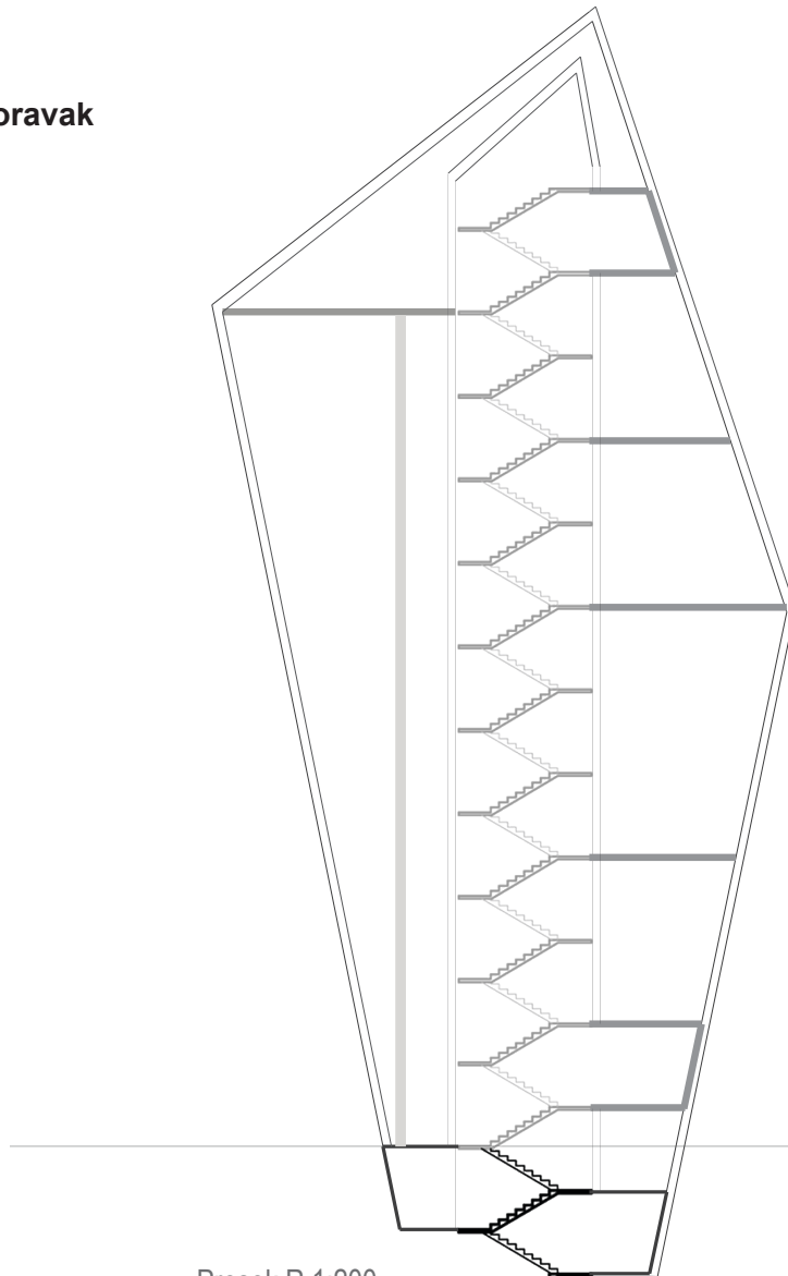
Presek R 1:200
