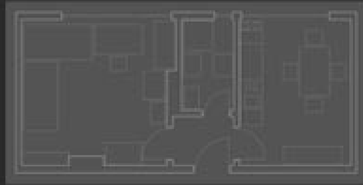
R=1:50 osnova stana-zatečeno stanje 2 korisnika
