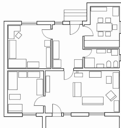
osnova postojećeg stanja r=1:200
