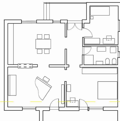
osnova redizajna r=1:200
