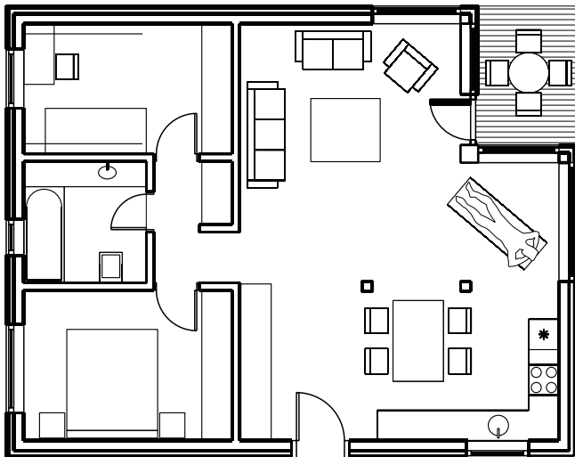
POSTOJA OSNOVA
