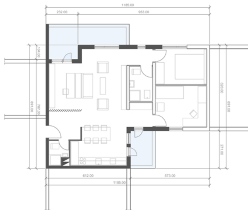
OSNOVA STANA-REKONSTRUKCIJA
