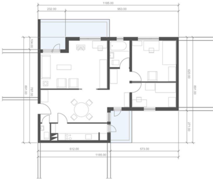
OSNOVA STANA-POSTOJEĆE STANJE
