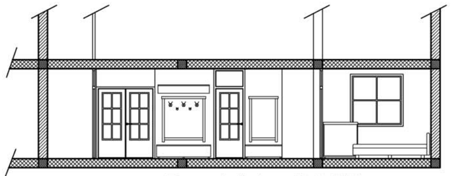
Presek 1-1 R 1:100
