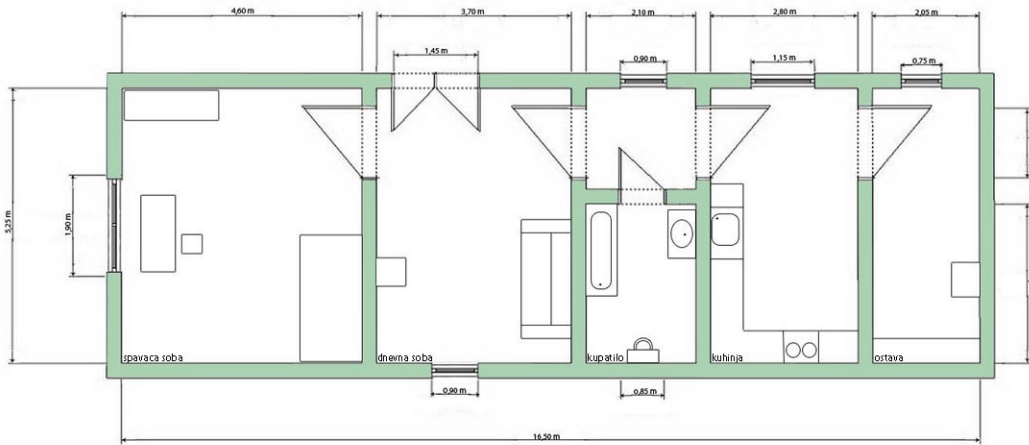
osnova stana - postojeće stanje R=1:50
