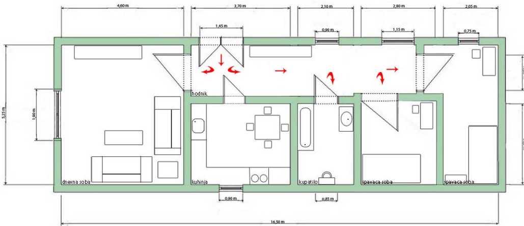
osnova stana - rekonstrukcija R=1:50
