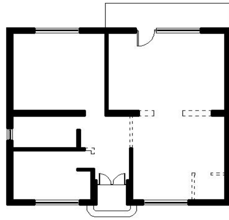
OSNOVA 2 R 1:100
