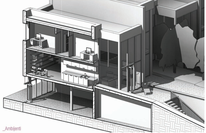
_3D presek stambeno poslovne jedinice
