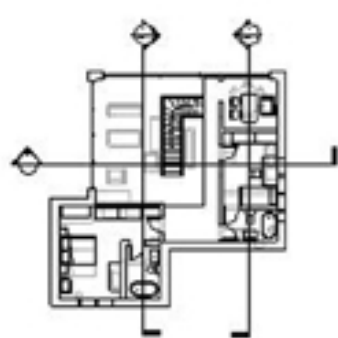
osnova sprata
