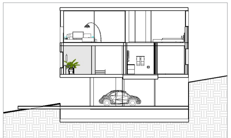
PRESEK 3-3
