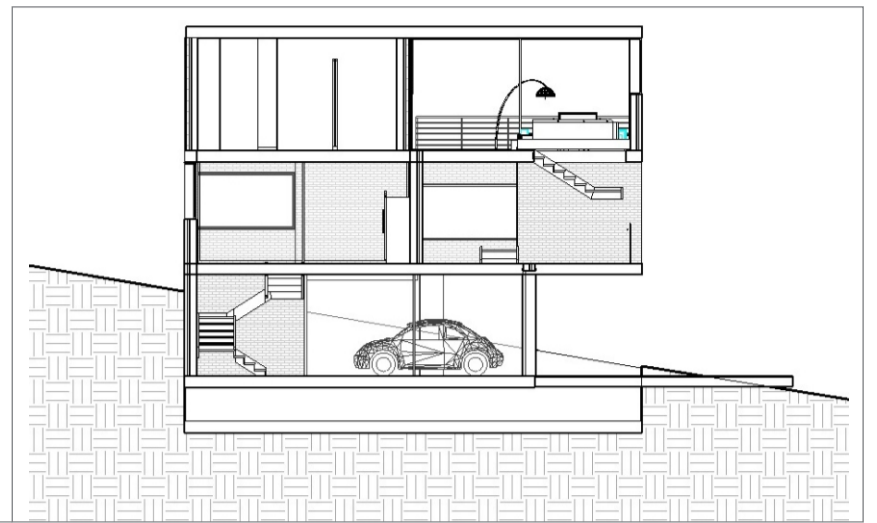
PRESEK 1-1
