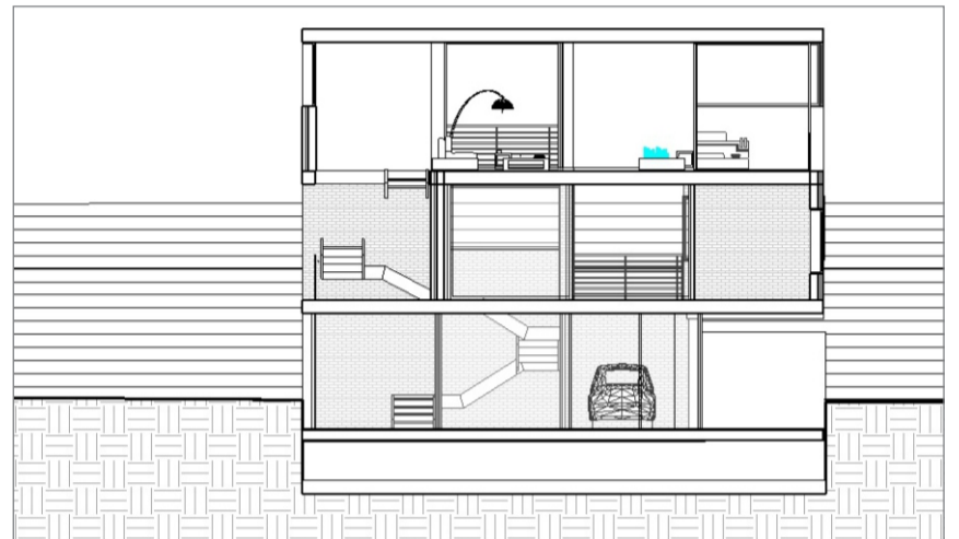
PRESEK 2-2
