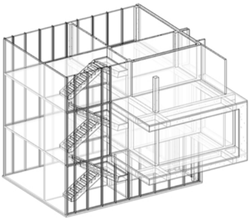
prikaz dela konstrukcije_3d view_section box hidden line_transparency 25
