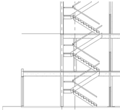
deo preseka
