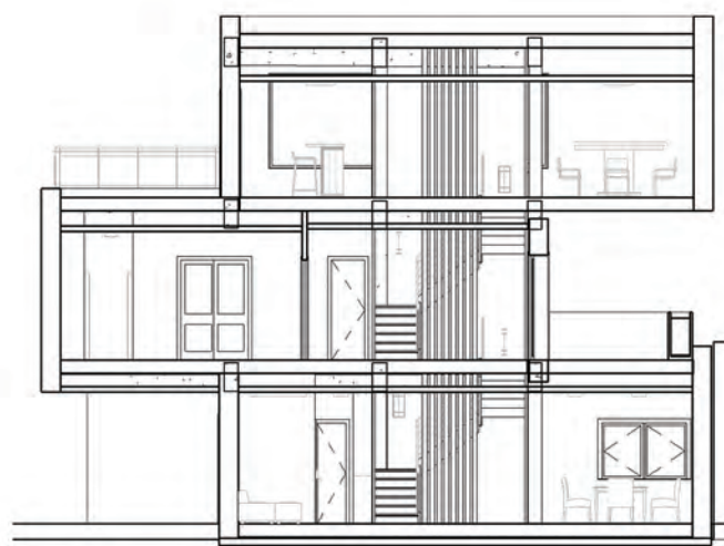
Presek 2-2
