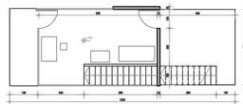
osnova drugog sprata R=1:200
