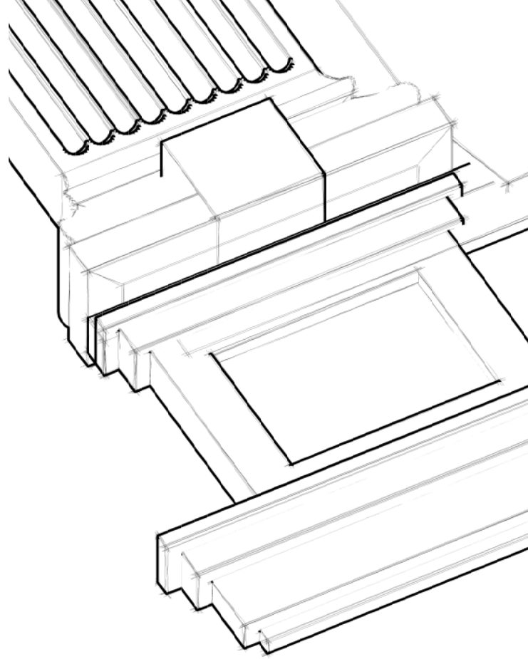
● detalj fasade
