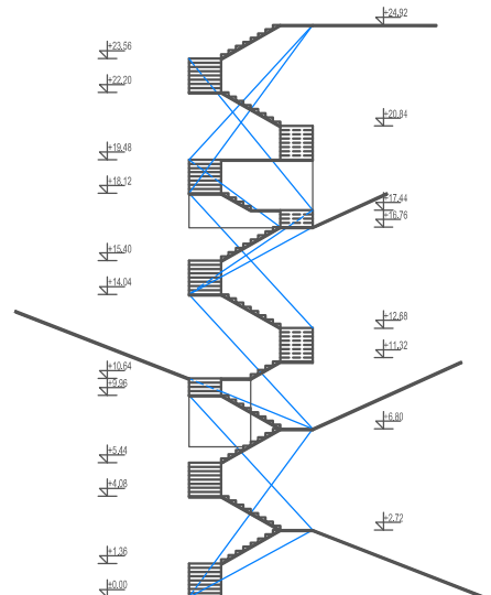
02 Presek A-A
