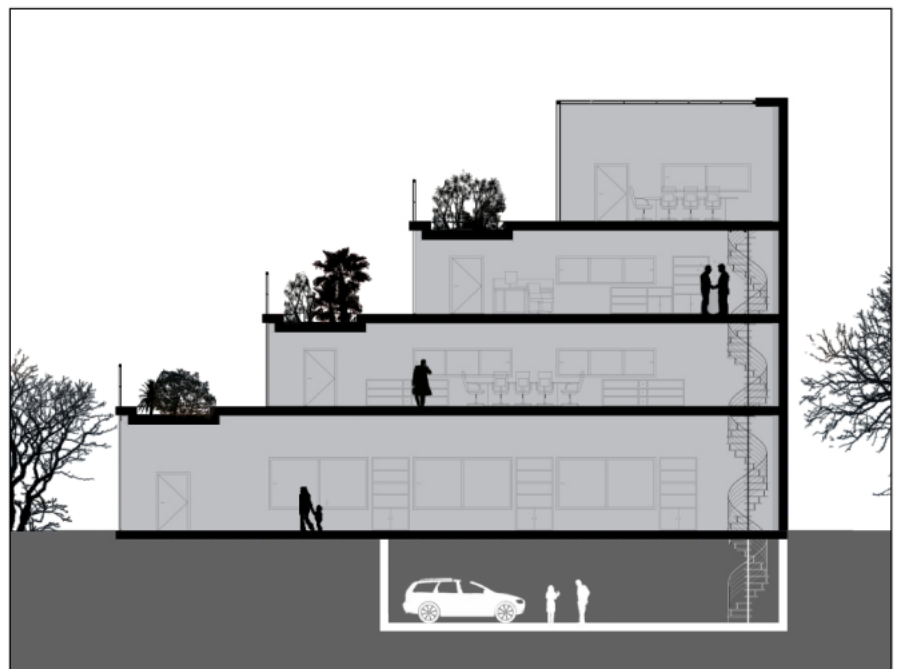
sl.3 presek kroz objekat
