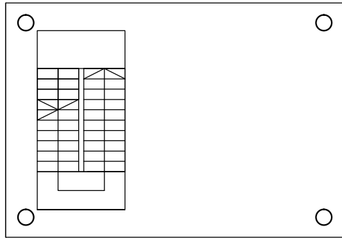
osnova partera
