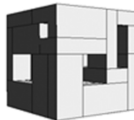
inicijalnih 27 kubusa dimenzija 1*2*4
