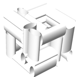
varijacija dobijena pomocu elipse
